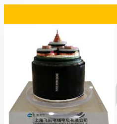
6~35kV电力电缆
